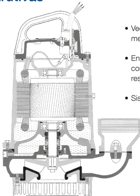
Imagem em corte de uma UNI 1000T
