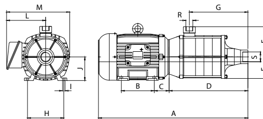
DIMENSÕES EM MILÍMETROS (mm) - 60 Hz
