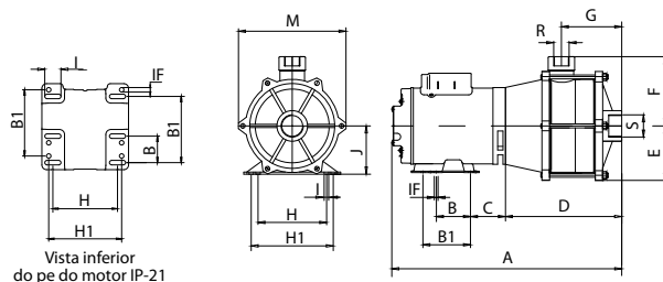
MOTOBOMBA IP-21
