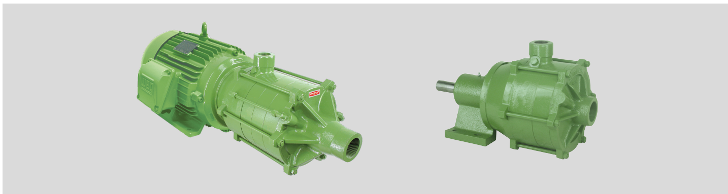
Motobombas de alta pressão, fornecidas com 2 a 7 estágios.
